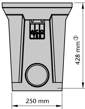
Optional riser
